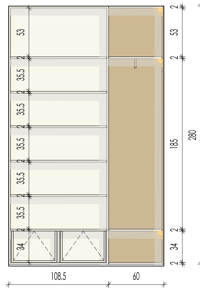
GARDEROBA DZIECI-WIDOK A-A | OTWARTA
