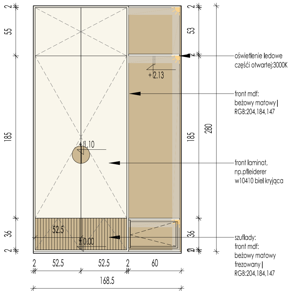
GARDEROBA DZIECI-WIDOK A-A | ZAMKNIĘTA
